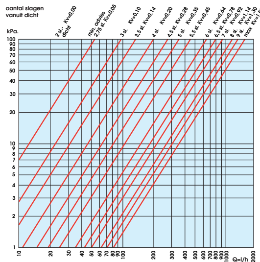
Drukverliesdiagram 2-pijps instelbaar
