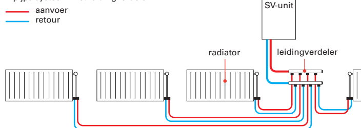
2-pijps systeem met leidingverdeler
